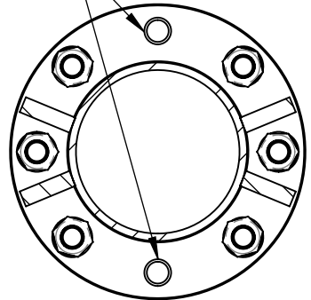
A-A (1 : 5) Anordnung der Flanschbolzen beachten! Check the arrangement of the flange bolts!
