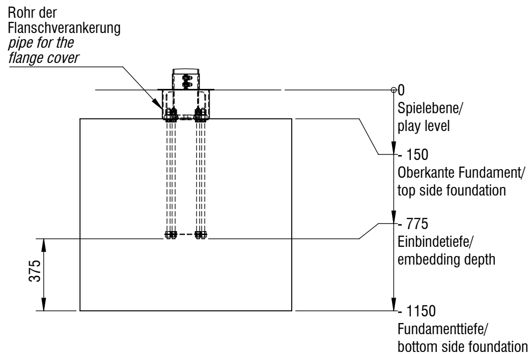
DETAIL Z (1 : 20)
