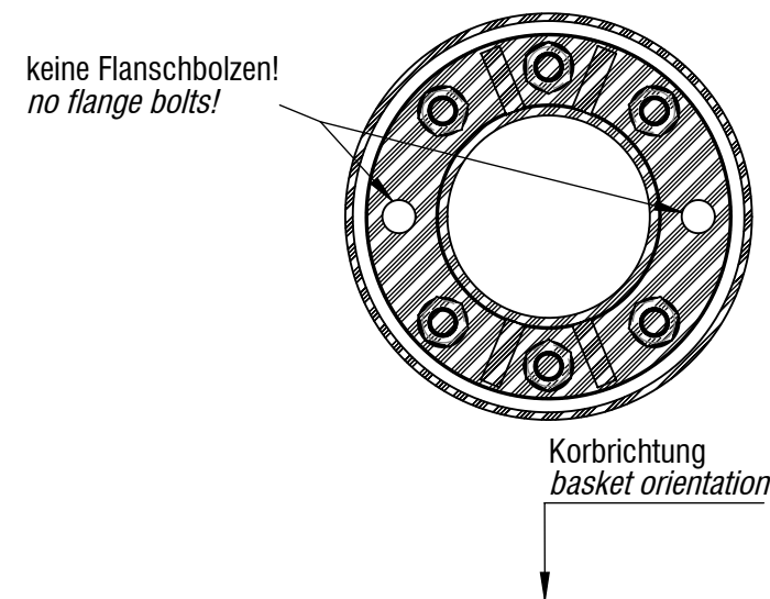
A-A (1 : 5) Anordnung der Flanschbolzen beachten! Check arrangement of the flange bolts!
