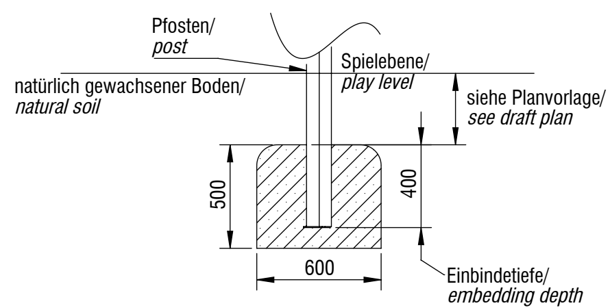
Fundamentschnitt Rutschenstützpfeilen/ foundation cut slide support post
