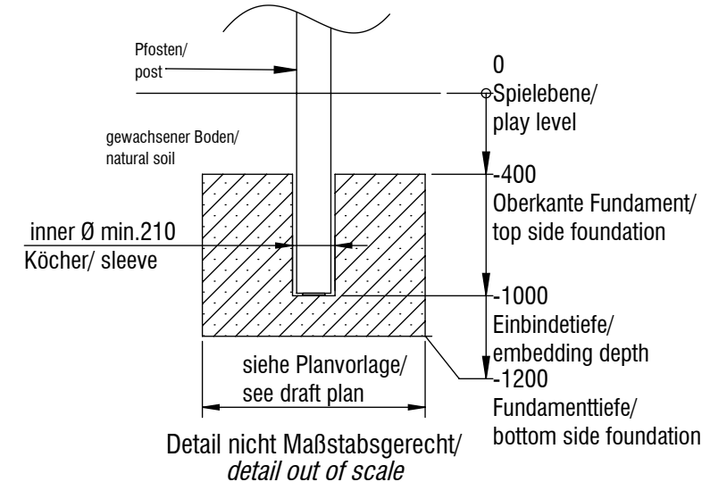
Fundamentschnitt Pfeilen/ foundation cut section post SP01
