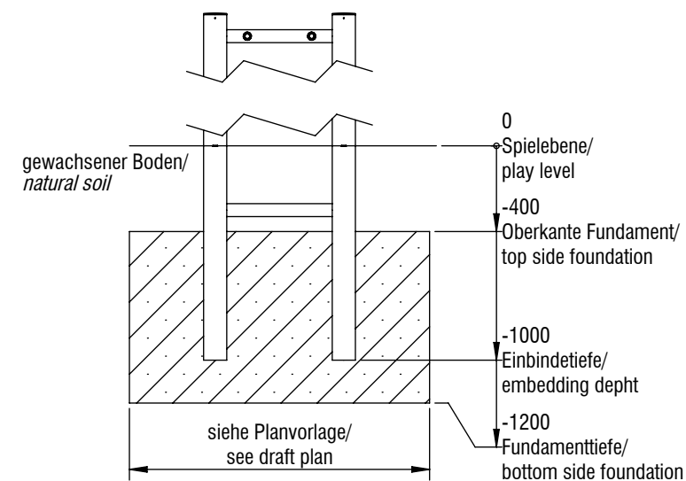
Fundamentschnitt H-Stütze / foundation cut H-entry post HS01 und HS02
