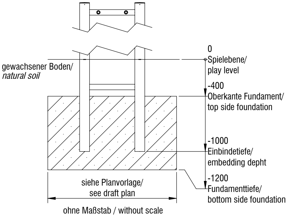
Fundamentschnitt H-Stütze / foundation cut H-support HS01
