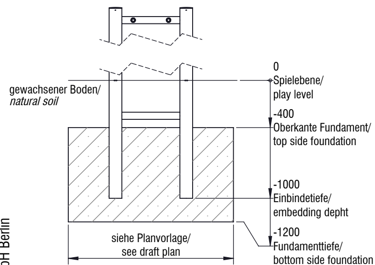
H - Stütze/ H - post HS01
