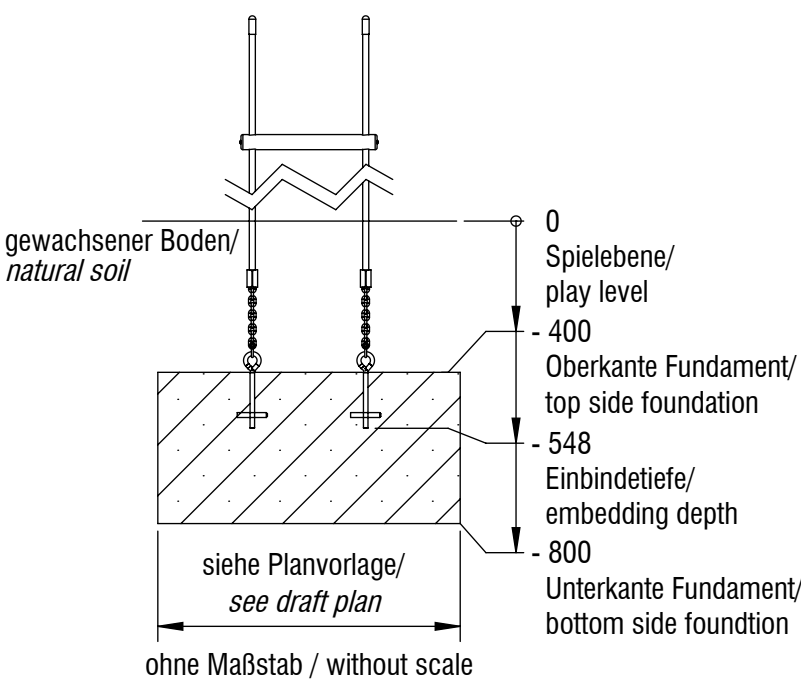
Fundamentschnitt Kletterleiter/ foundation cut climbin ladder
