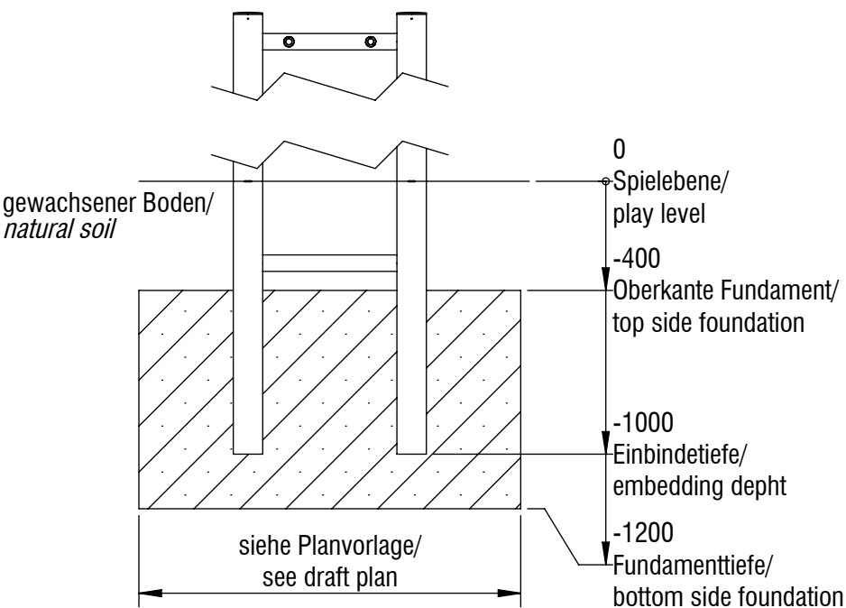
Fundamentschnitt H-Stütze/ foundation cut h-support HS01
