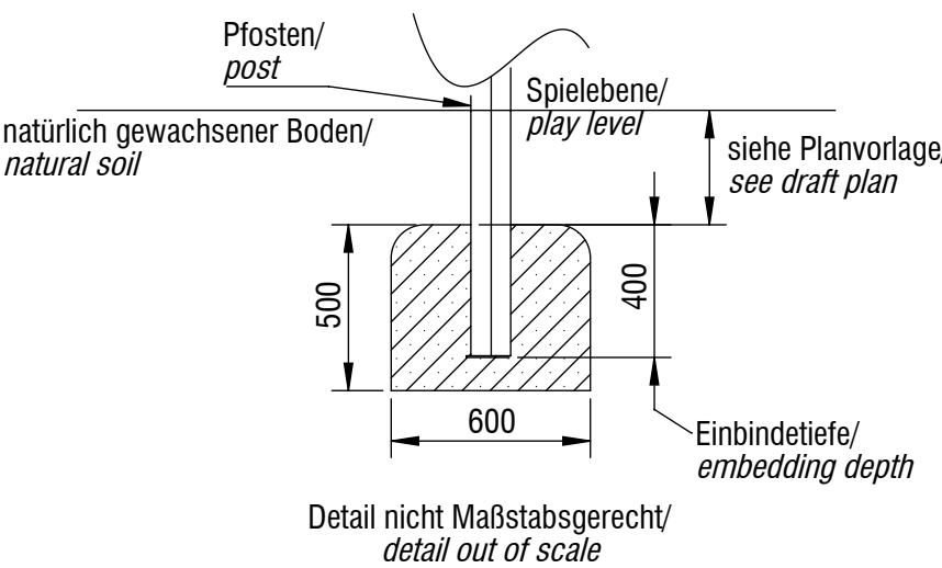
Fundamentschnitt Rutschenstützpfoften/ foundation cut slide support post
