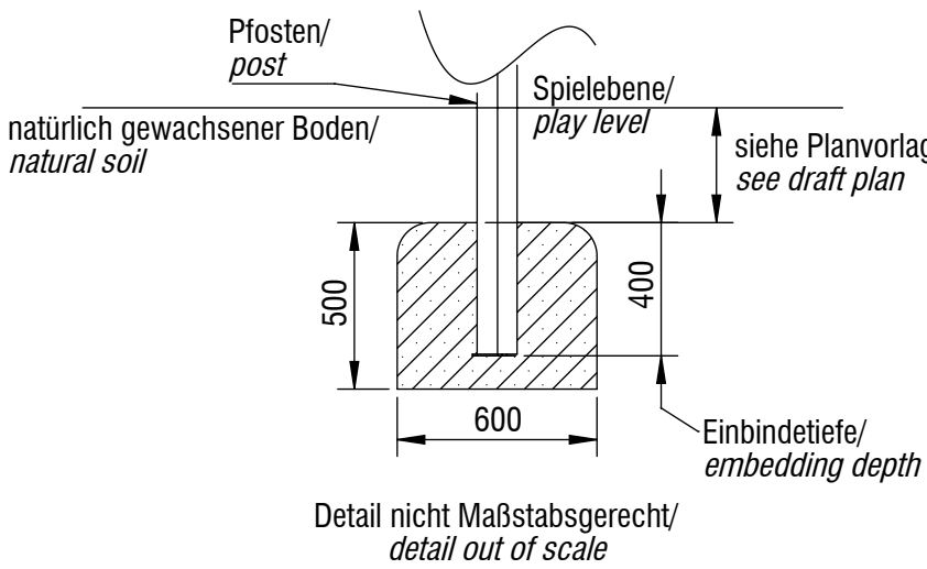
Fundamentschnitt Rutschenstützpfeiler/ foundation cut slide support post
