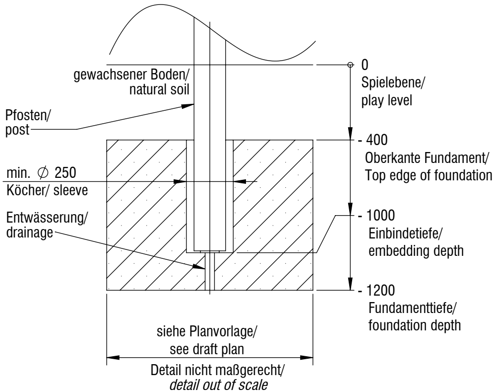
Fundamentschnitt Rutschenstützpfeiler/ foundation cut slide support post
