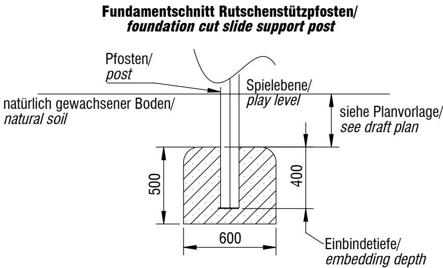
Detail nicht Maßstabsgerecht/ detail out of scale
