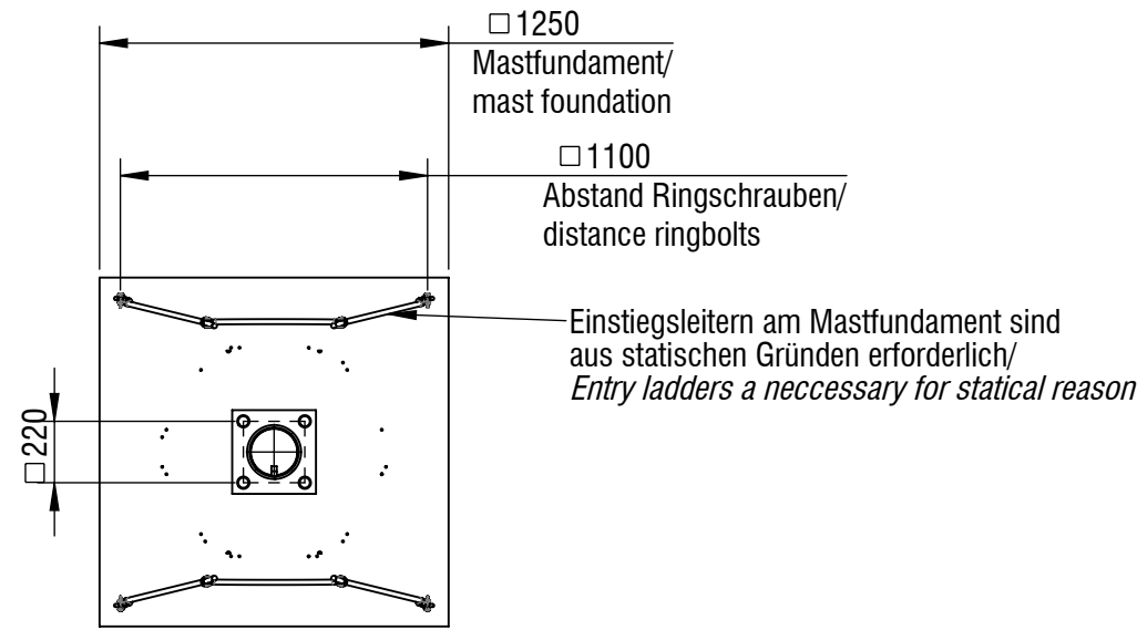
DETAIL A MAßSTAB: 1 : 30
