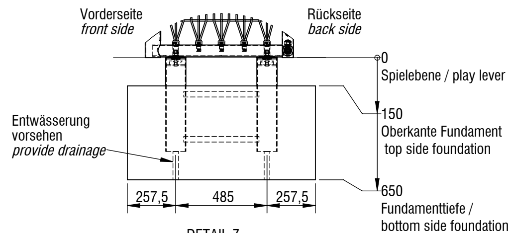
DETAIL Z MAßSTAB: 1 : 20 Fundamentdetail foundation detail citytor original
