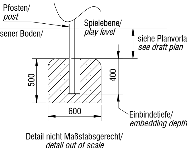
Fundamentschnitt Rutschenstützpfosten/ foundation cut slide support post
