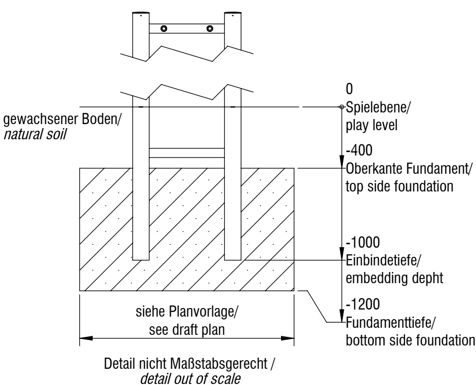
Fundamentschnitt H-Stütze HS01 / foundation cut H-post HS01
