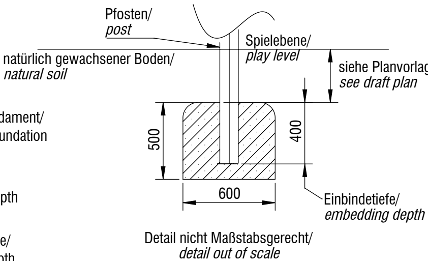
Fundamentschnitt Rutschenstützpfosten/ foundation cut slide support post
