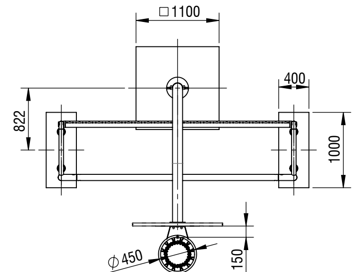
A-A (1 : 5) Anordnung der Flanschbolzen beachten! Check the arrangement of the flange bolts!
