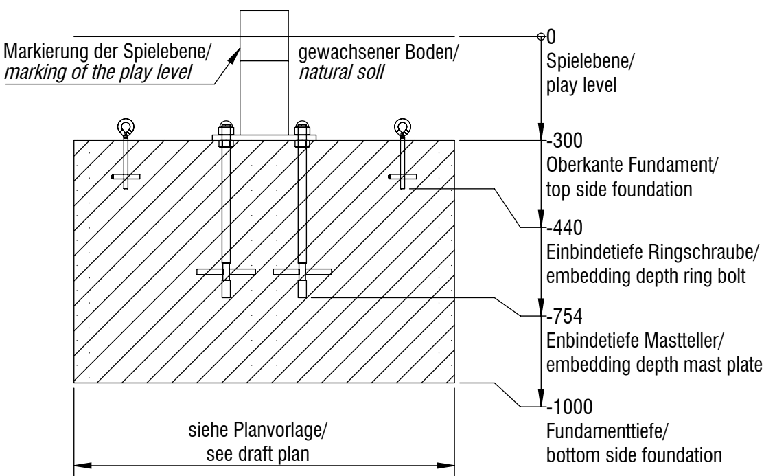
Fundamentschnitt/ foundation cut Mastteller im Mastfundament/ mast plate in mast foundation
