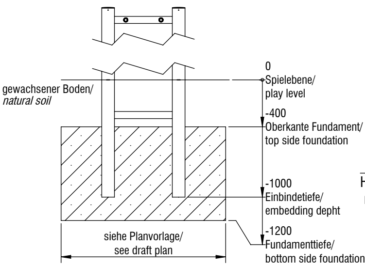
Fundamentschnitt H-Stütze/ foundation cut H-support
