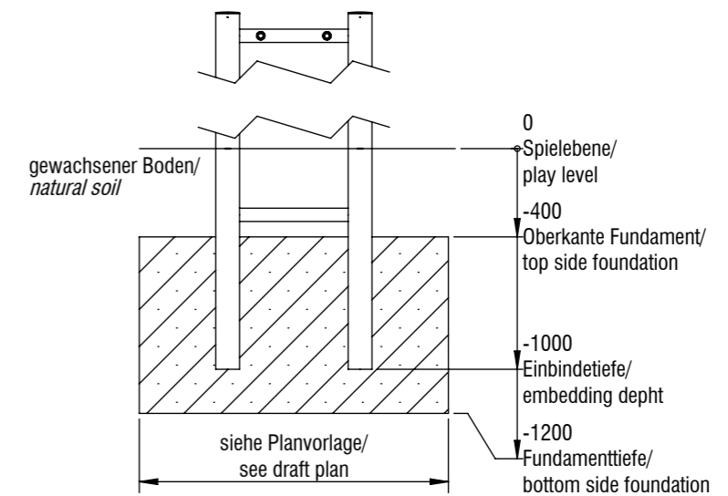
Fundamentschnitt H-Stütze/ foundation cut H-support
