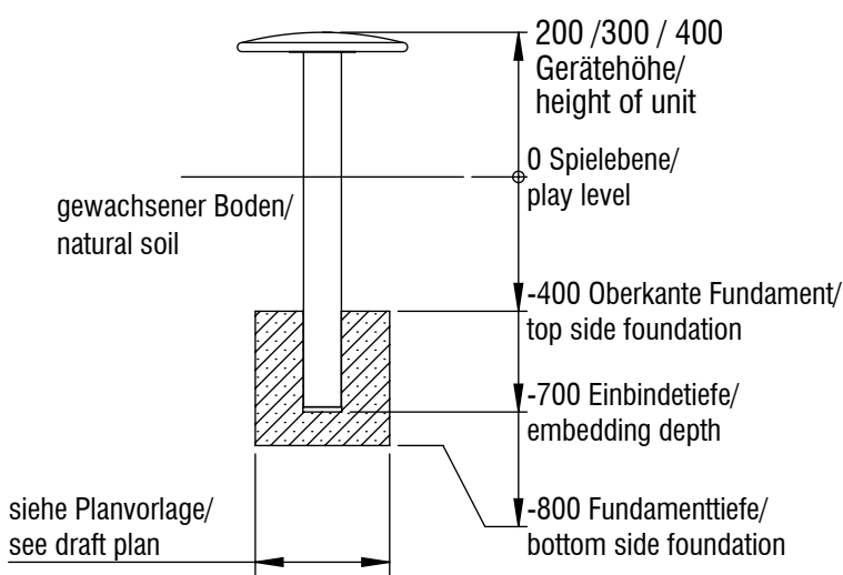
Detail nicht maßstabsgerecht/ detail out of scale
