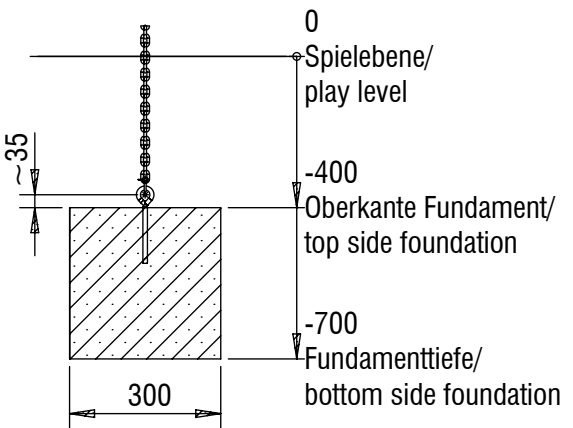
Detail nicht maßstabsgerecht/ detail out of scale
