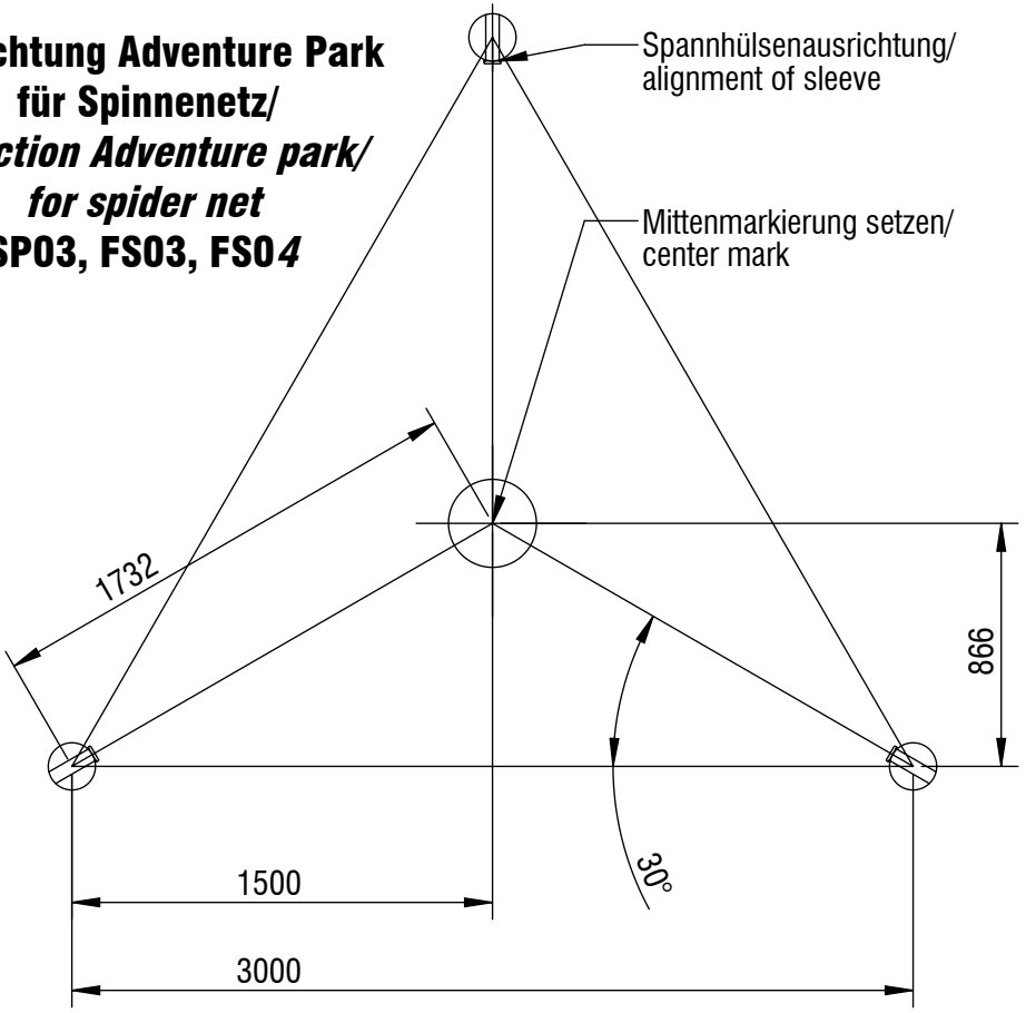
Detail nicht maßstabsgerecht/ detail out of scale
