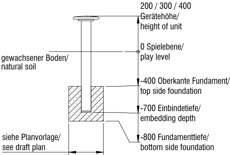
Detail nicht maßstabsgerecht/ detail out of scale
