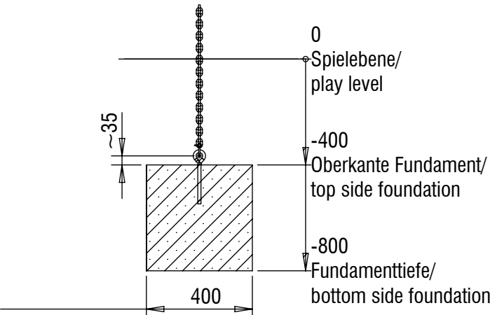
Detail nicht maßstabsgerecht/ detail out of scale
