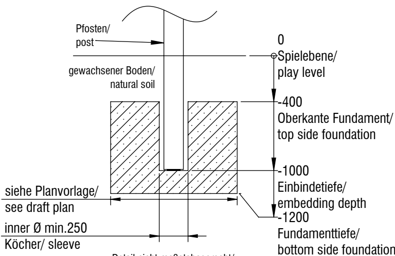
Detail nicht maßstabsgerecht/ detail out of scale
