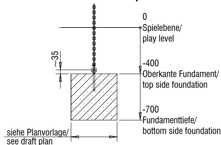
Fundamentschnitt Regentropfen/ foundation cut raindrops
