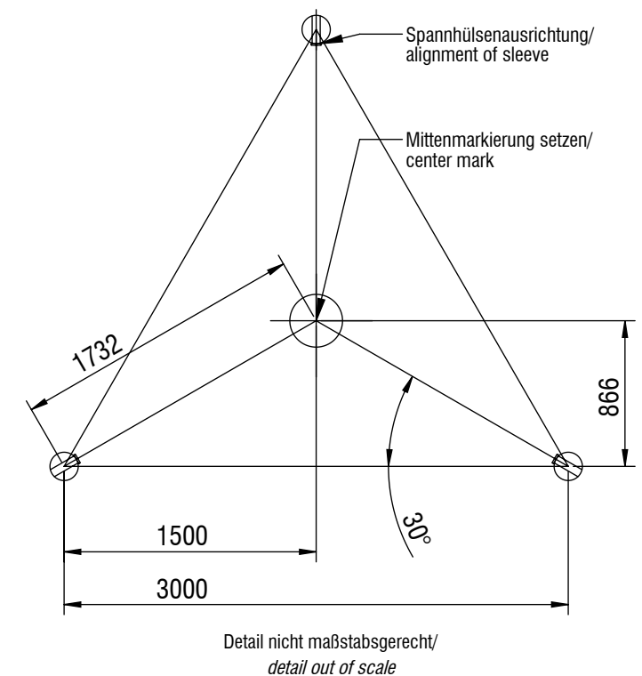
Ausrichtung Spinnenhöhle und Dschungel Lounge/ alignment of spider cave and jungle lounge
