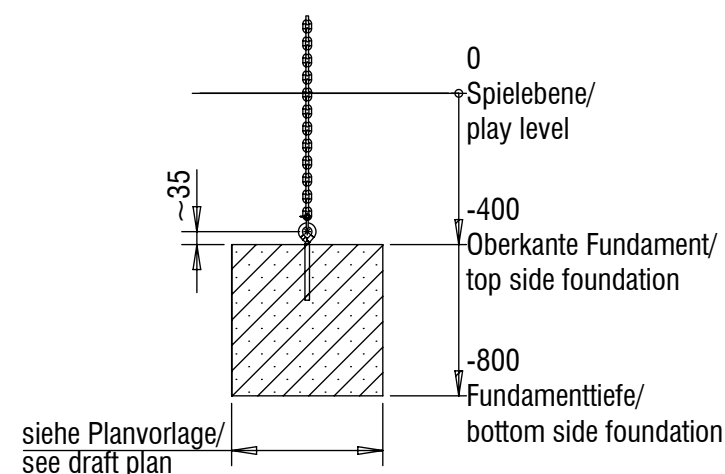
Fundamentschnitt Lianenpark/ foundation cut liana park
