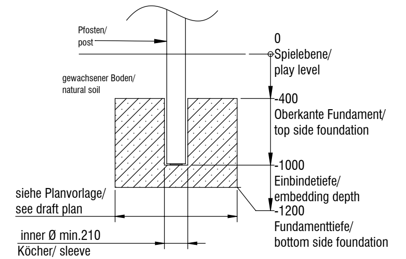
Fundamentschnitt Pfosten/ foundation cut SP01 - SP15
