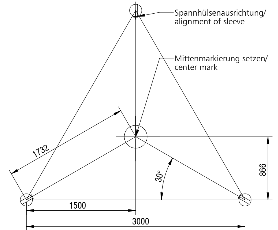
Ausrichtung Spinnenhöhle und Dschungel Lounge/ alignment of spider cave and jungle lounge
