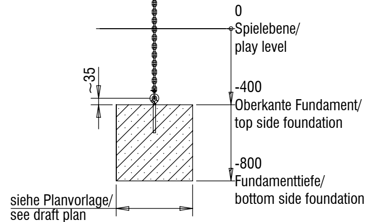
Fundamentschnitt Regentropfen/ foundation cut raindrops
