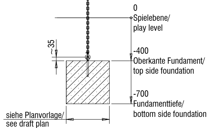
Fundamentschnitt Lianenpark/ foundation cut liana park
