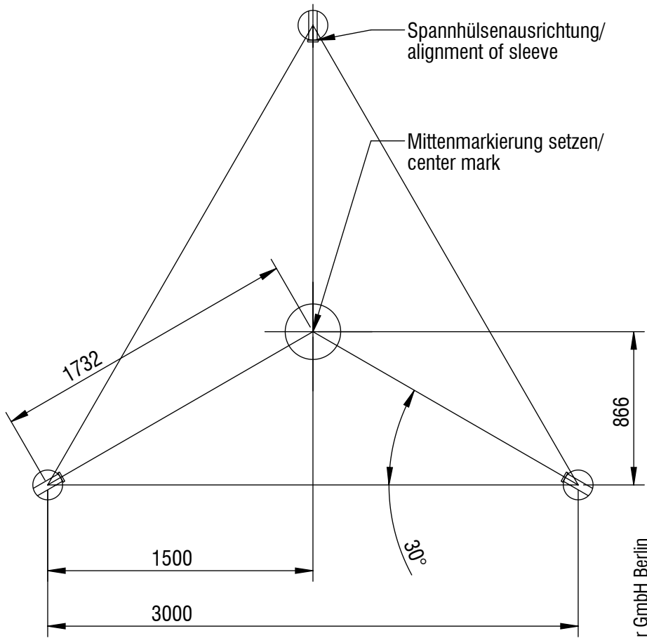
Ausrichtung Spannhülsen bei der Dschungel Lounge Alignment of sleeves for the Jungle Lounge
