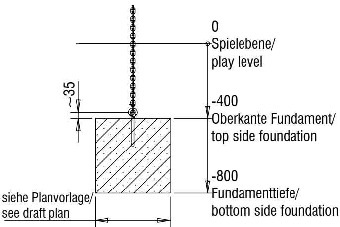
Fundamentschnitt Lianenpark/ foundation cut liana park
