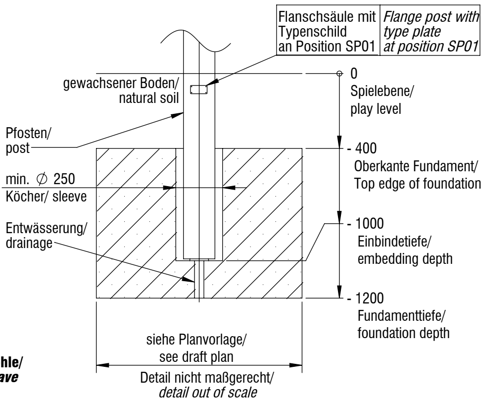
Fundamentschnitt Pfosten/ foundation cut SP01 - SP09
