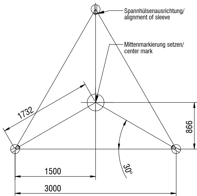
Ausrichtung Spinnenhöhle/ alignment of spider cave
