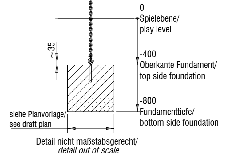
Fundamentschnitt Lianenpark/ foundation cut liana park
