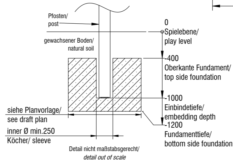
Fundamentschnitt Pfosten/ foundation cut SP01 - SP09
