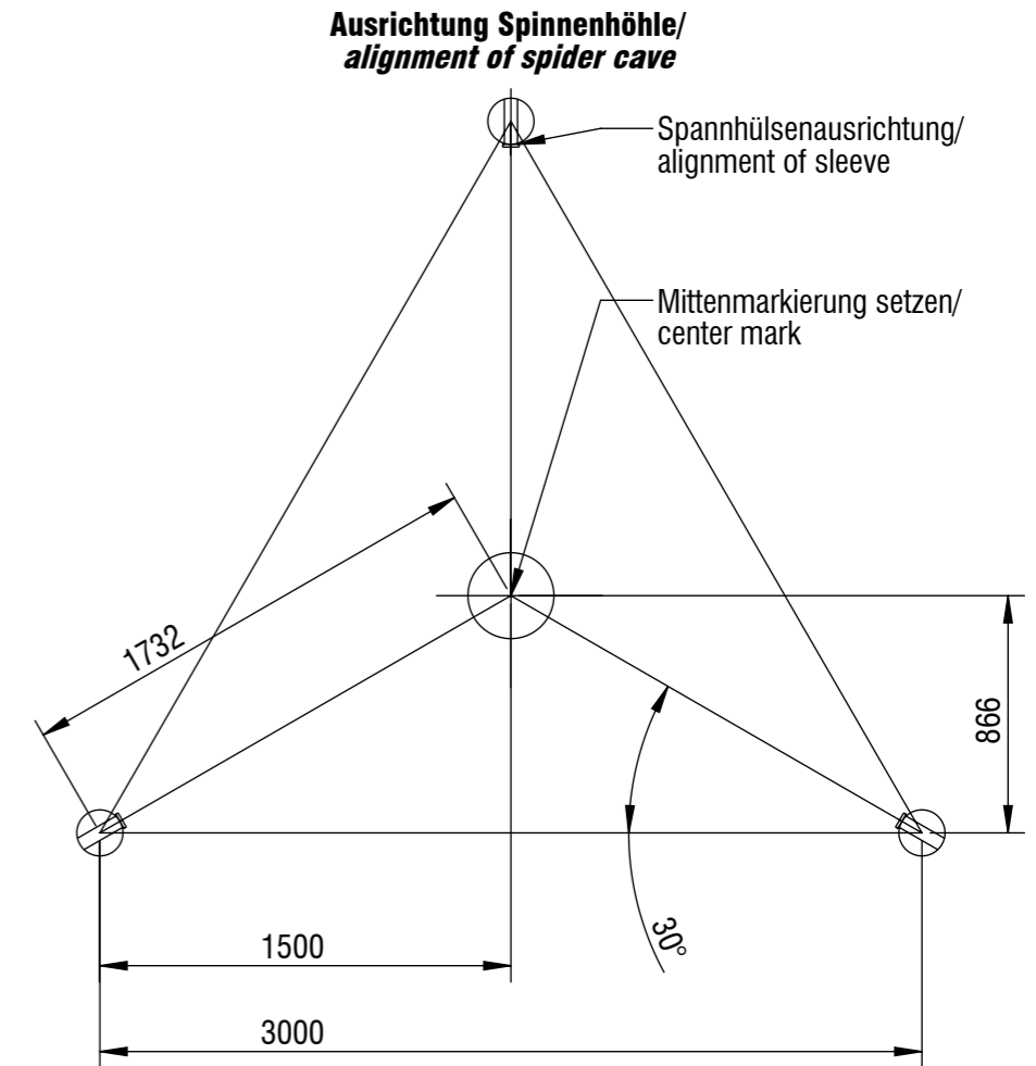
Detail nicht maßstabsgerecht/ detail out of scale
