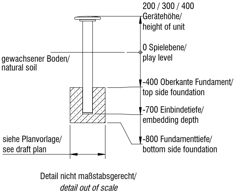
Fundamentschnitt Kleiner Käfer/ foundation cut Big beetle FS03, FS04
