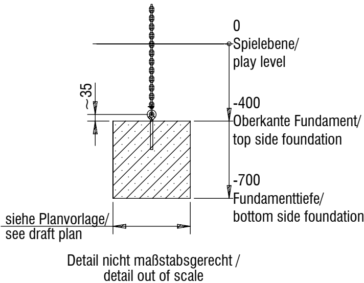
Fundamentschnitt Regentropfen/ foundation cut raindrops
