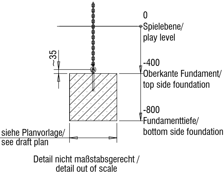
Fundamentschnitt Lianenpark/ foundation cut liana park
