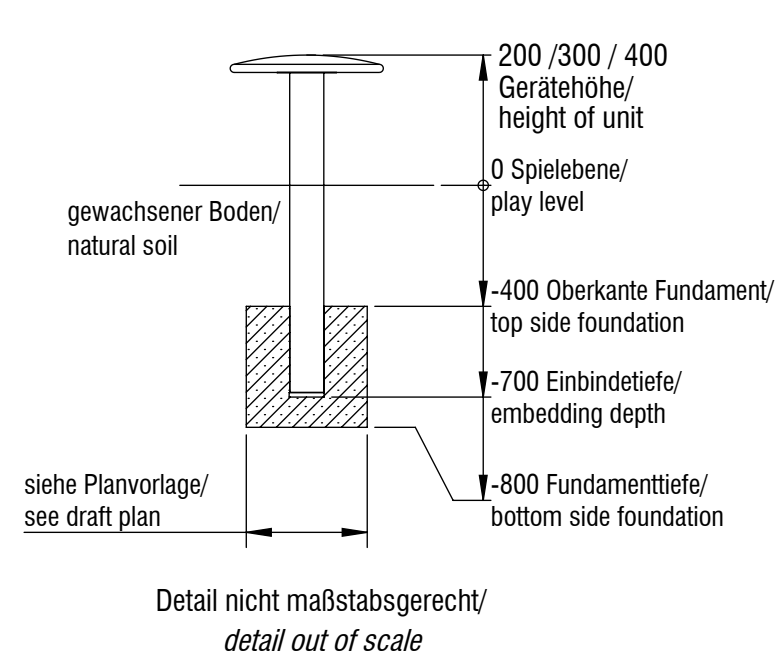
Fundamentschnitt Großer Käfer/ foundation cut Big beetle FS02
