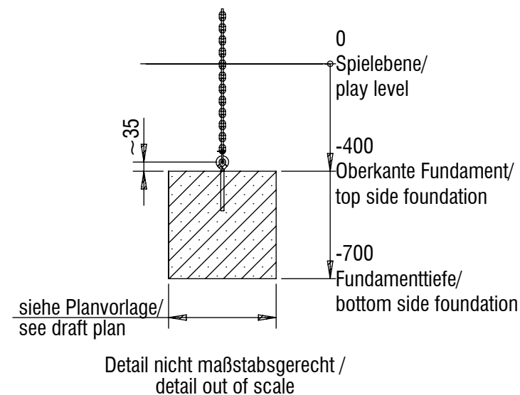
Fundamentschnitt Regentropfen/ foundation cut raindrops
