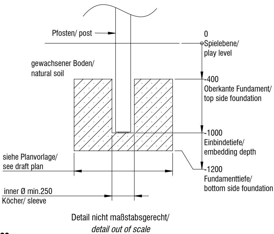
Fundamentschnitt Pfosten / foundation cut SP01-SP06
