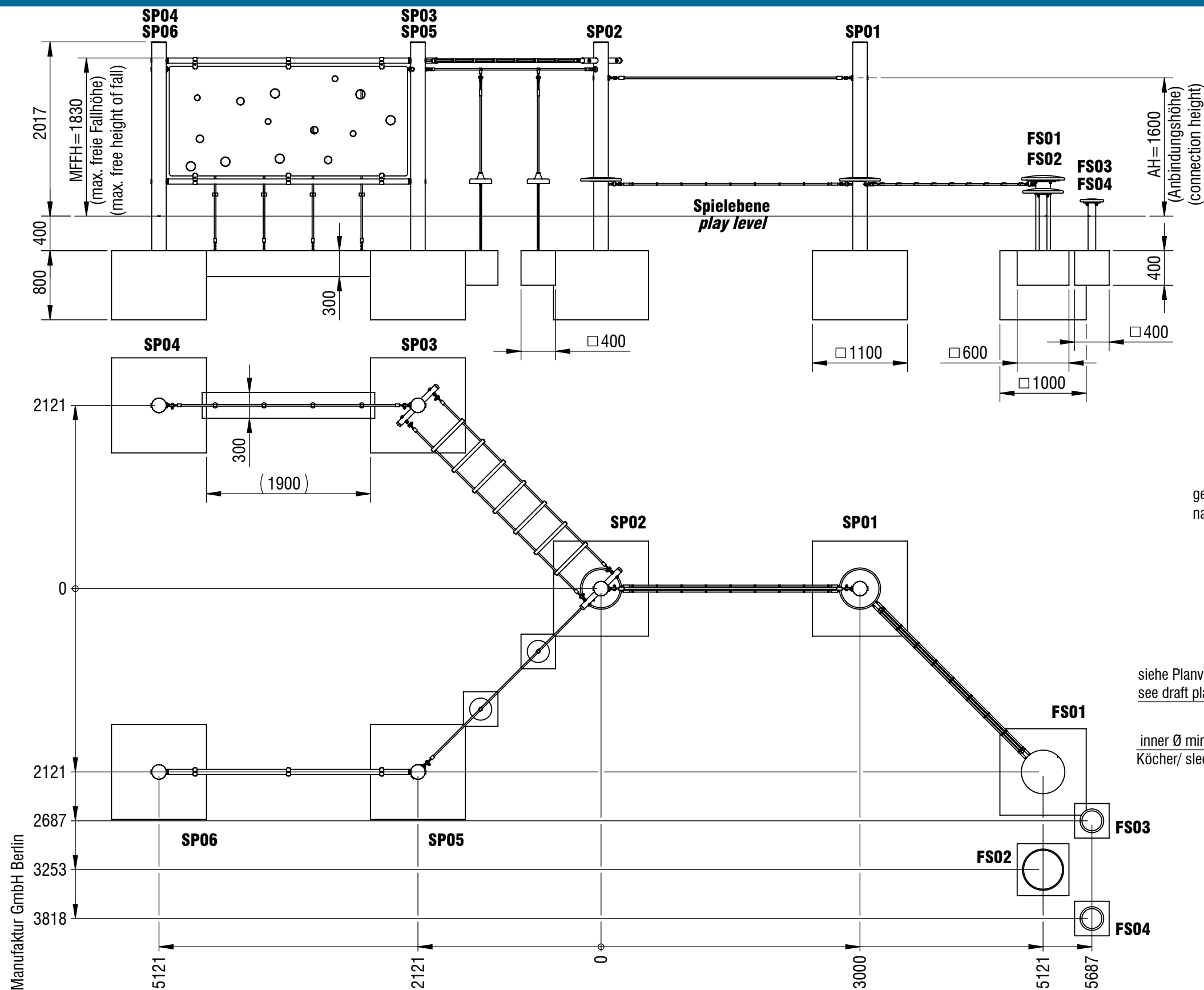
Fundamentschnitt Pfosten / foundation cut SP01-SP06
