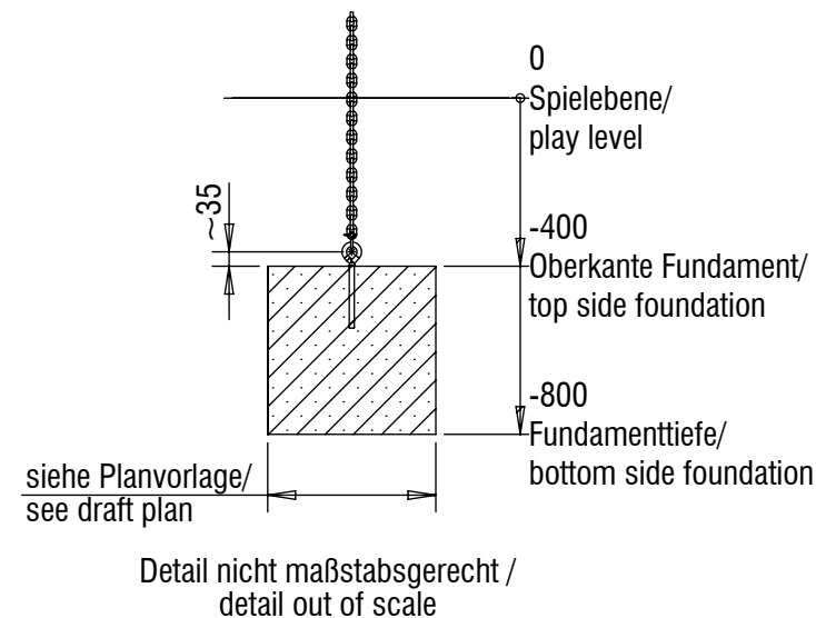
Fundamentschnitt Lianenpark/ foundation cut liana park
