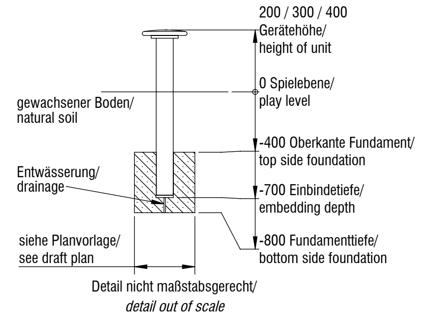
Fundamentschnitt Kleiner Käfer / foundation cut small beetle FS01
