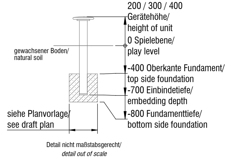
Fundamentschnitt Kleiner Käfer / foundation cut small beetle FS01
