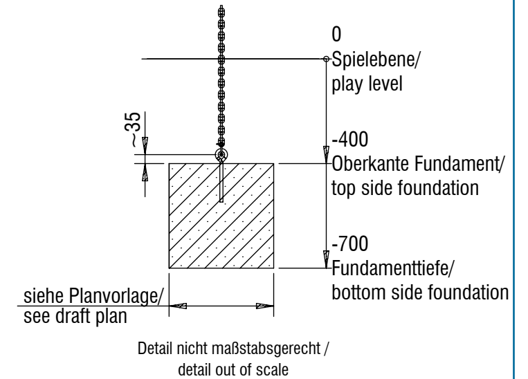
Fundamentschnitt Regentropfen/ foundation raindrops SP03-SP04
