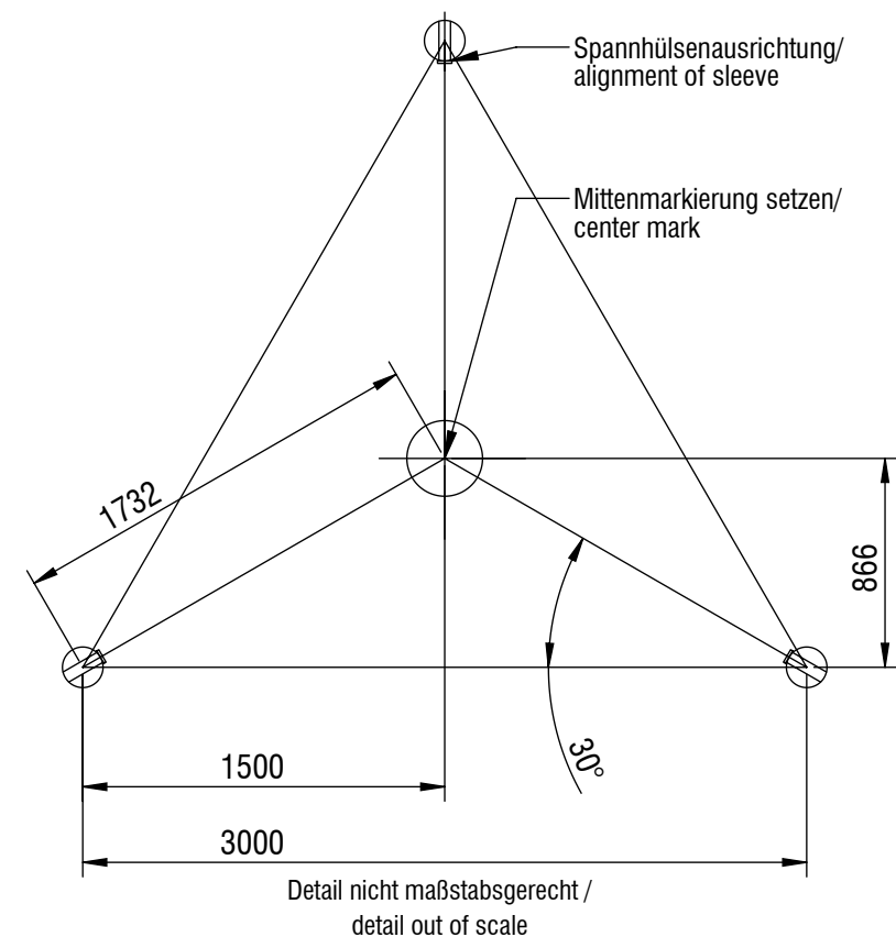
Ausrichtung Stützpfeiler Spinnenhöhle / alignment support post Spider cave
