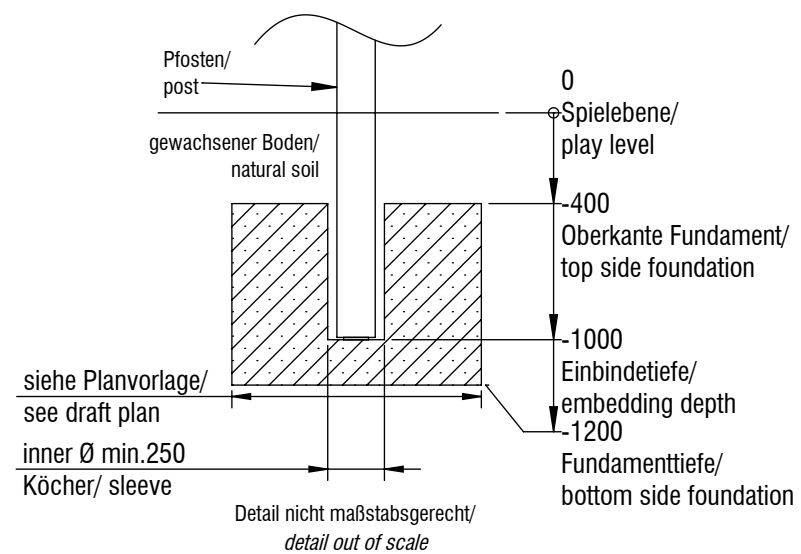
Fundamentschnitt Pfosten/ foundation cut SP01-SP06
