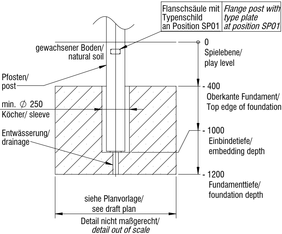
Fundamentschnitt FS01 / foundation cut FS01
