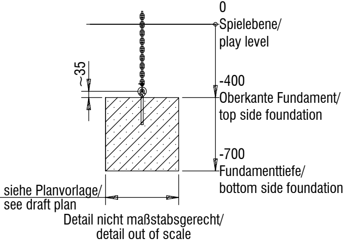
Fundamentschnitt Regentropfen / foundation cut raindrop
