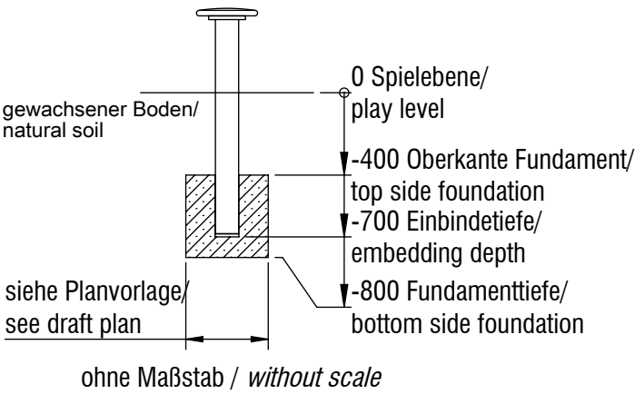
Fundamentschnitt kleiner Käfer/ foundation cut small beetle
