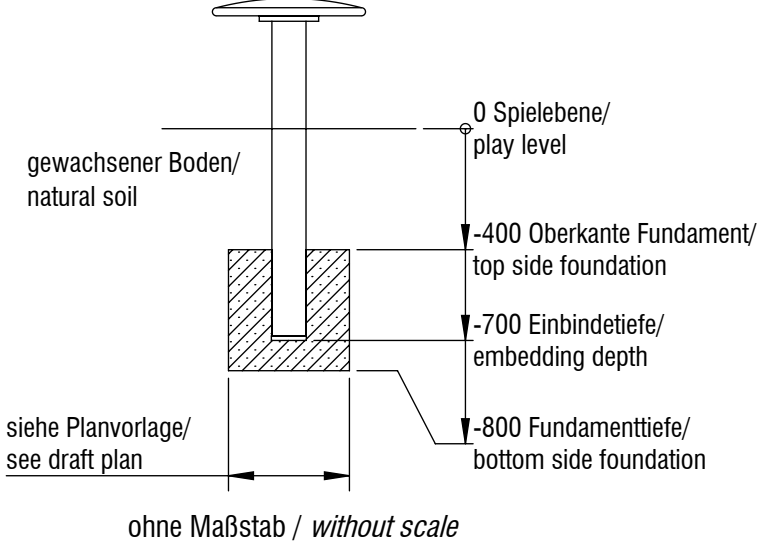
Fundamentschnitt großer Käfer/ foundation cut big beetle
