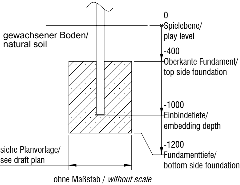
Fundamentschnitt Pfosten/ foundation cut post
