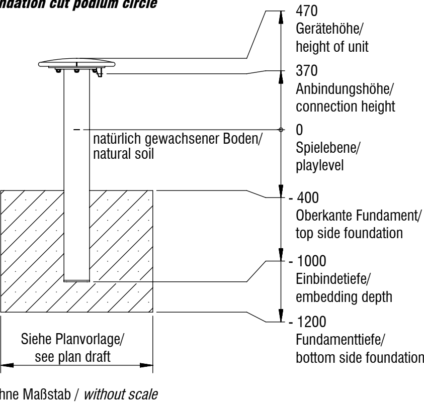
Fundamentschnitt Podium circle/ foundation cut podium circle
