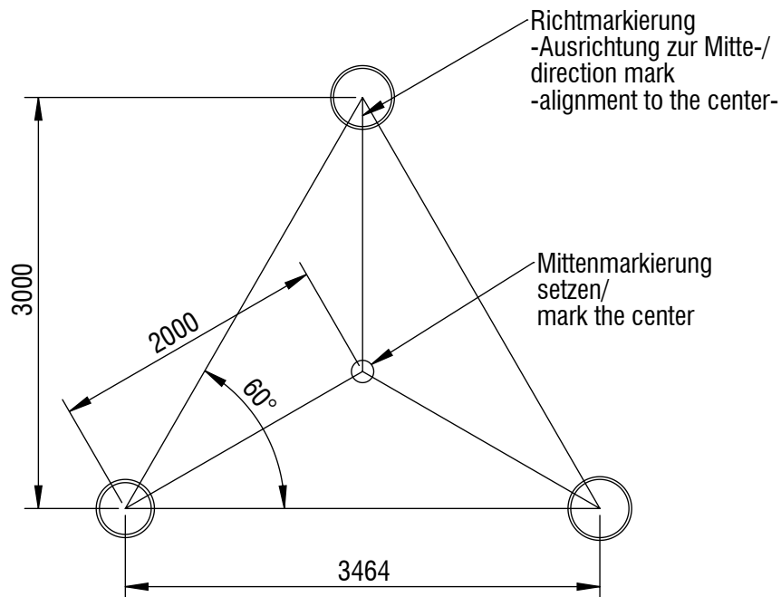
Ausrichtung Schwebebänder / alignment for ropeway Flux 02, Flux 03
