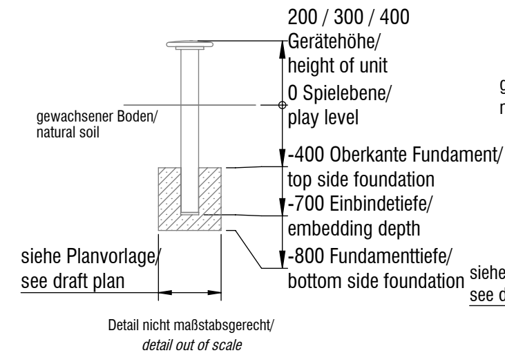
Fundamentschnitt Kleiner Käfer / foundation cut Small beetle FS01, FS03, FS04, FS06
