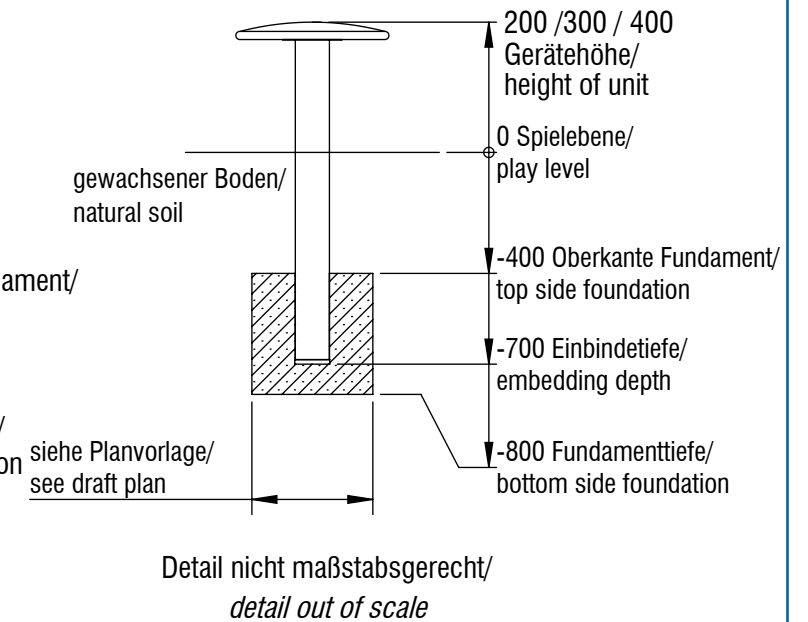
Fundamentschnitt Großer Käfer / foundation cut Big beetle FS02, FS05
