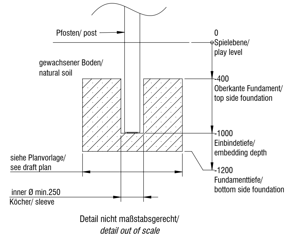
Fundamentschnitt Pfosten / foundation cut SP01 - SP06
