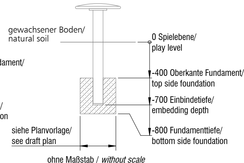
Fundamentalschnitt Großer Käfer / foundation cut Big beetle FS02, FS05
