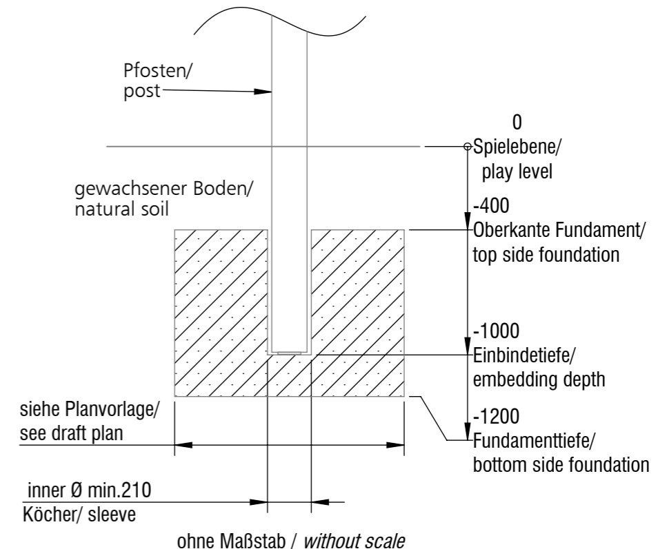
Fundamentalschnitt Pfosten / foundation cut SP01 - SP06
