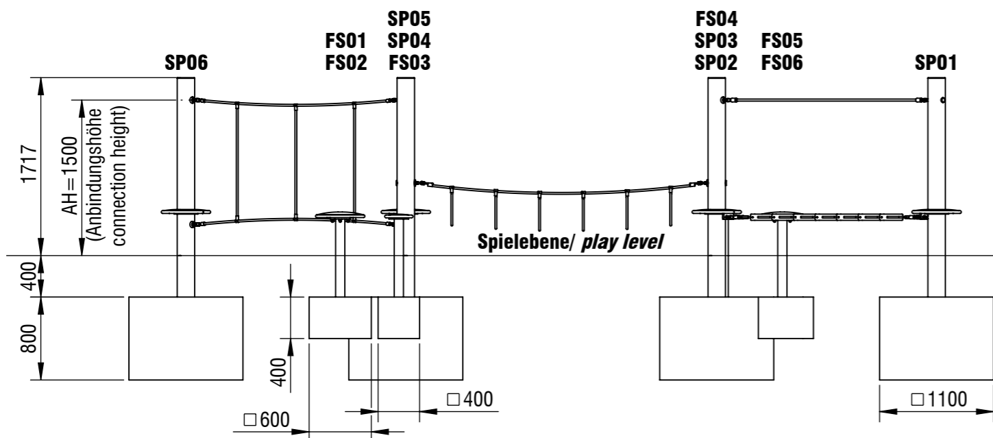
Fundamentalschnitt Kleiner Käfer / foundation cut Small beetle FS01, FS03, FS04, FS06
