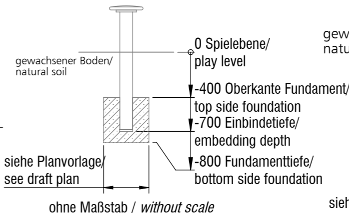
Fundamentalschnitt Kleiner Käfer / foundation cut Small beetle FS01, FS03, FS04, FS06
