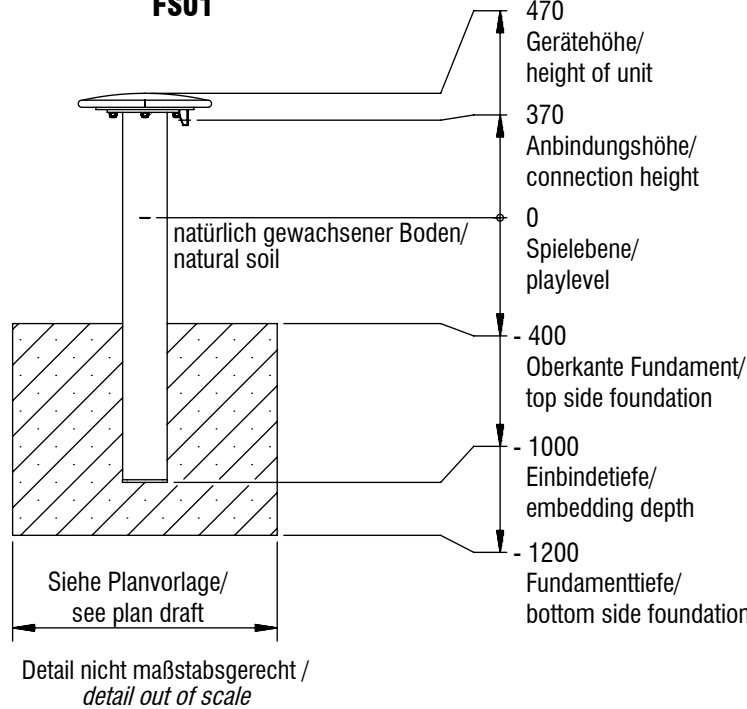
Fundamentschnitt Flanschsäule/ foundation cut flang post FS01
