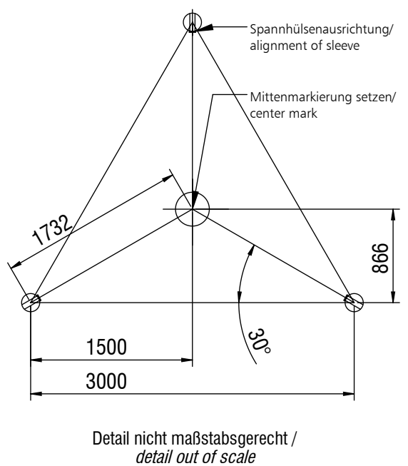
Ausrichtung der Pfosten für Orchideenblatt/ alignment for orchidea leaf posts SP01,SP03,SP04
