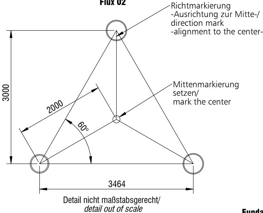
Ausrichtung Schwebebänder / alignment for ropeway Flux 02
