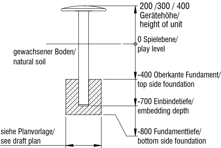
Fundamentschnitt großer Käfer/ foundation cut big beetle FS08 und FS17
