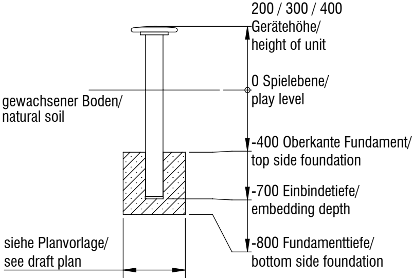
Fundamentschnitt kleiner Käfer/ foundation cut small beetle FS01- FS03,FS05- FS07,FS09-FS11,FS14-FS16, FS18-FS20 und FS22-FS24
