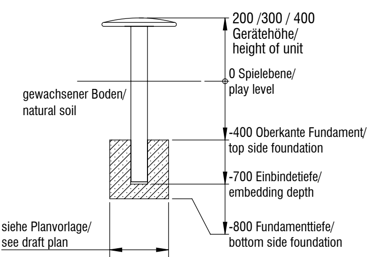
Fundamentschnitt großer Käfer/ foundation cut big beetle
