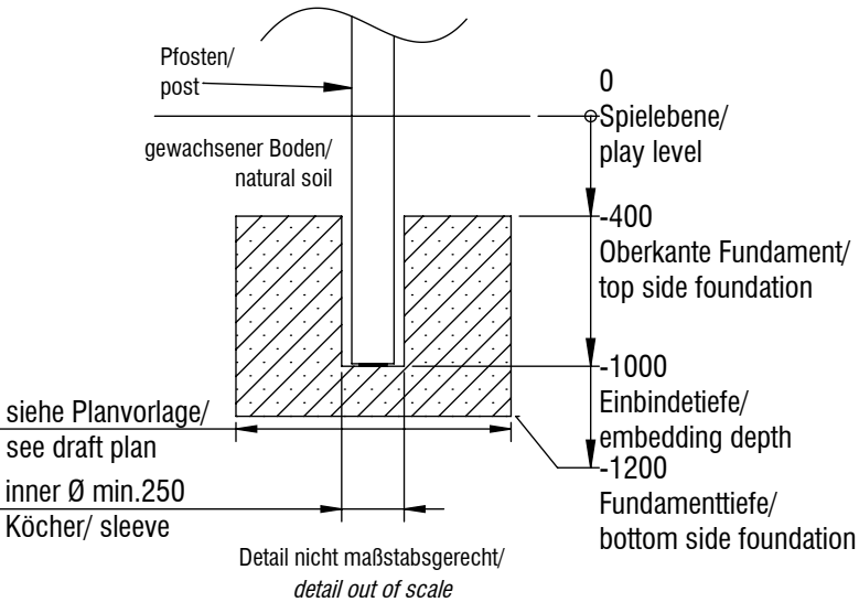
Fundamentschnitt Pfosten/ foundation cut post
