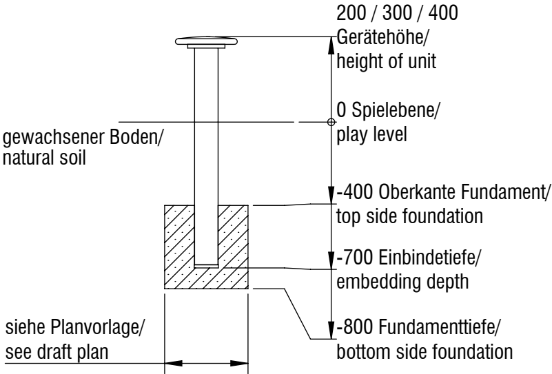
Fundamentschnitt kleiner Käfer/ foundation cut small beetle
