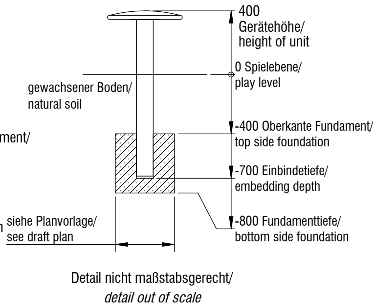
Fundamentschnitt Großer Käfer / foundation cut Big beetle FS02, FS05
