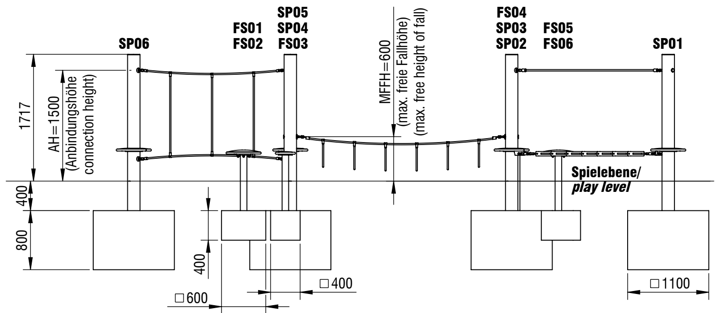
Fundamentschnitt Kleiner Käfer / foundation cut Small beetle FS01, FS03, FS04, FS06
