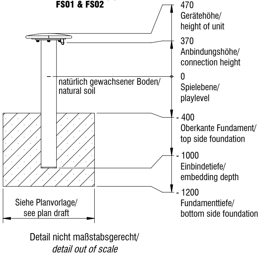
Fundamentschnitt Lianenpark/ foundation cut liana park
