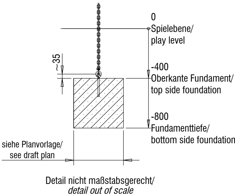
Fundamentschnitt Lianenpark/ foundation cut liana park
