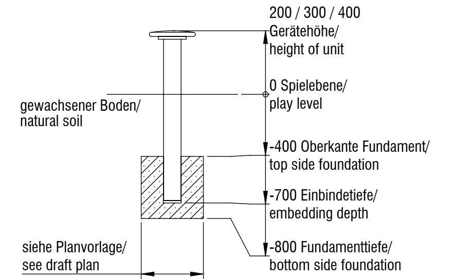
Fundamentschnitt kleiner Käfer/ foundation cut small beetle FS03 & FS04
