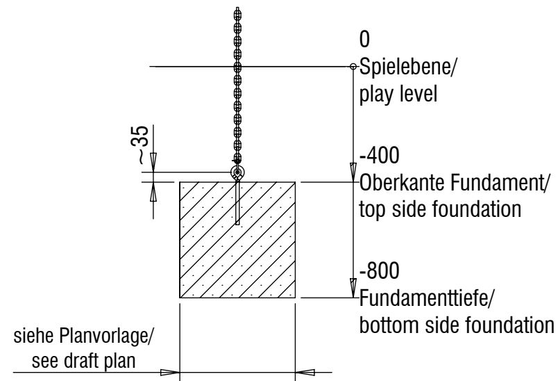
Fundamentschnitt Lianenpark/ foundation cut liana park
