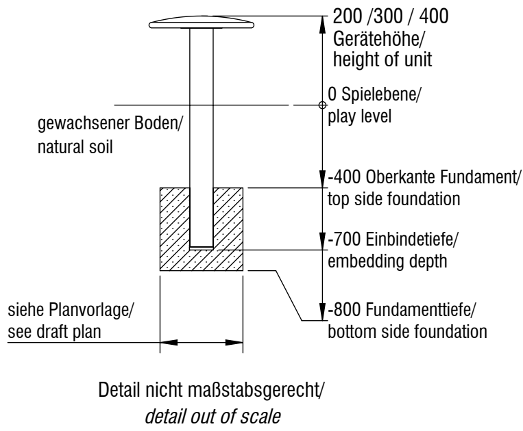
Fundamentschnitt Großer Käfer/ foundation cut big beetle FS03
