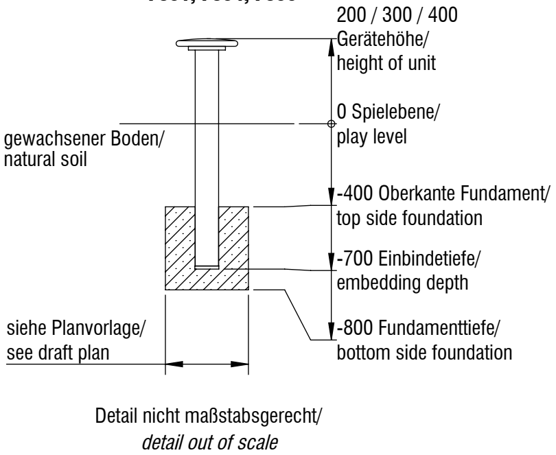
Fundamentschnitt Kleiner Käfer/ foundation cut small beetle FS01, FS04, FS05
